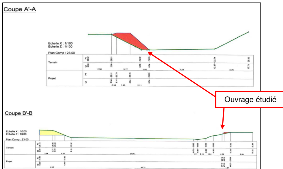
Extrait des coupes transversales du projet - INGETEC-02/06/2017
