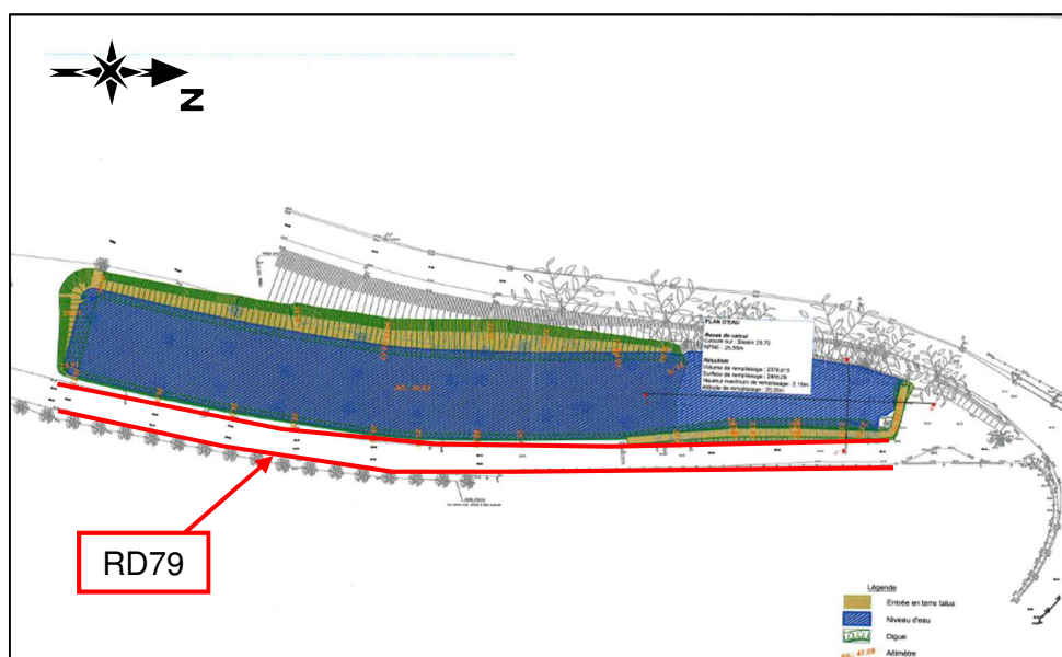
Extrait de la vue en plan –INGETEC-02/06/2017
