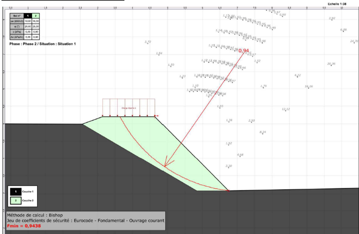
Résultat de calcul de stabilité en phase provisoire avec le logiciel TALREN (pente 1H/1V)
