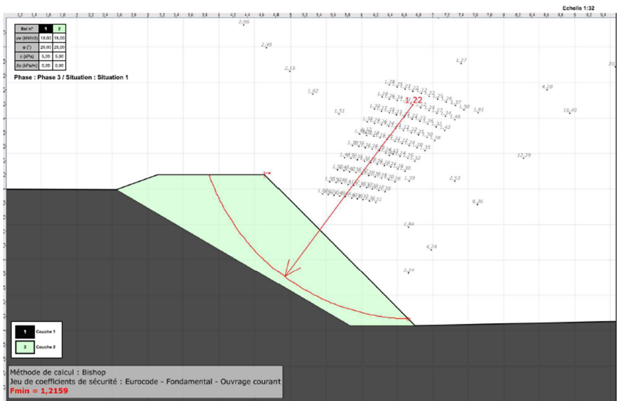
Résultat de calcul de stabilité en phase définitive avec le logiciel TALREN (pente 1H/1V)
